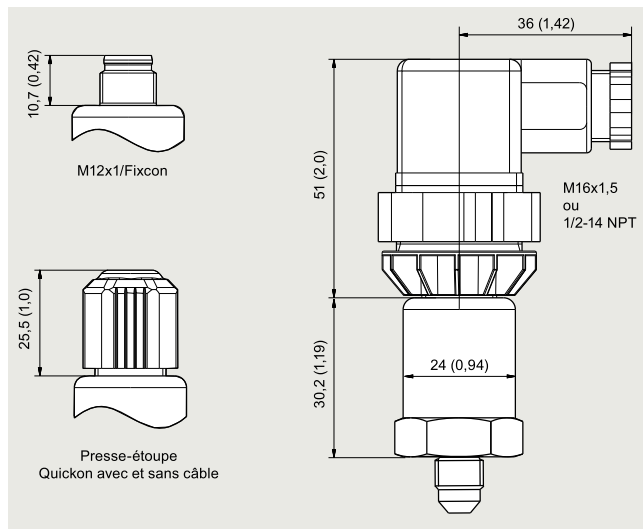
SITRANS P210, raccords électriques, dimensions en mm (pouces)
