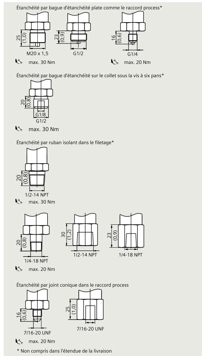
SITRANS P210, raccords process, dimensions en mm (pouces)
