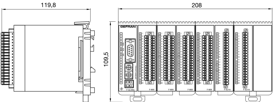
I/O 8 SLOT
