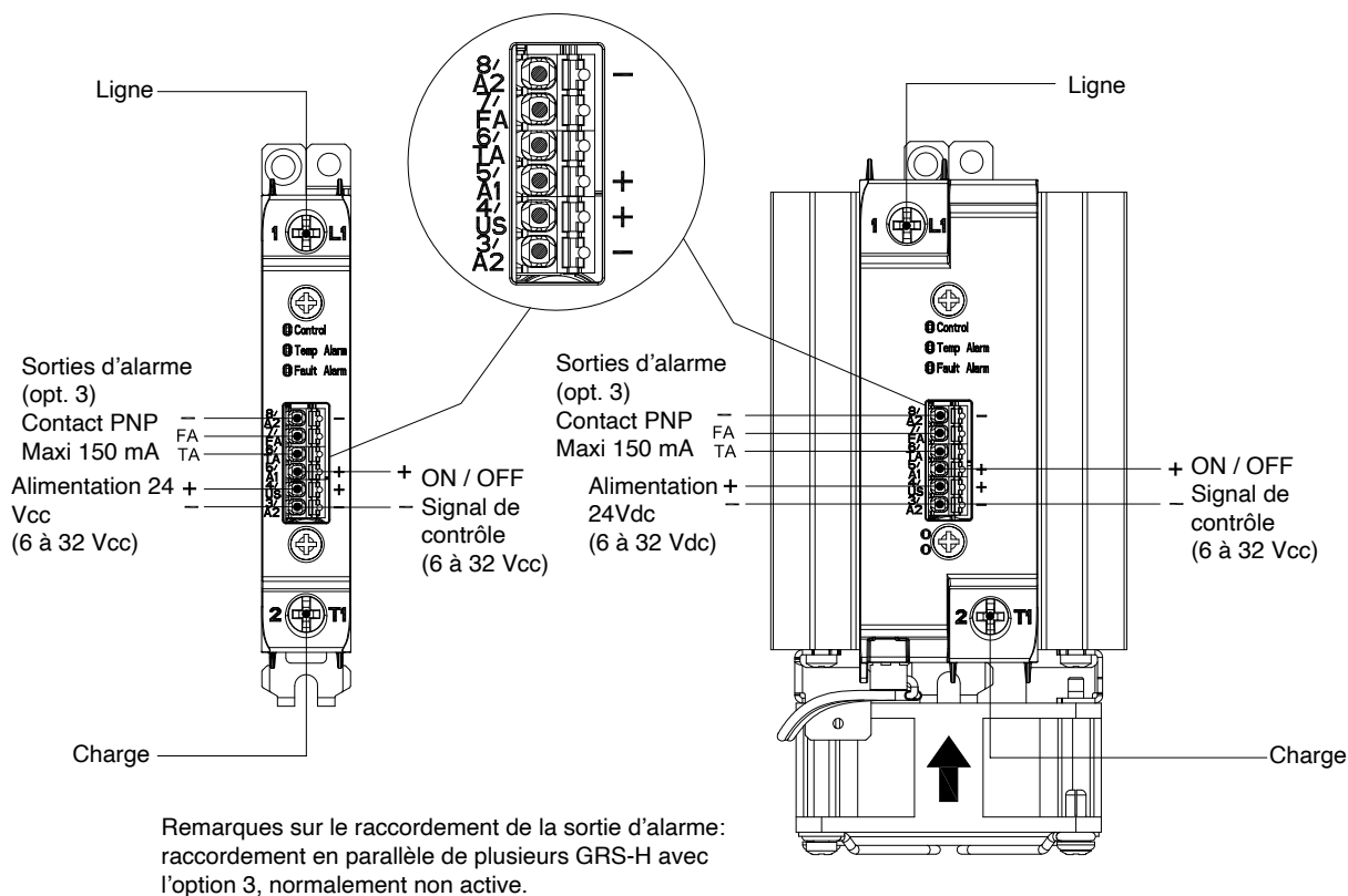
Exemple de raccordement pour GRS-H avec commande Vcc avec option de sortie d'alarme PNP (Option 3)
