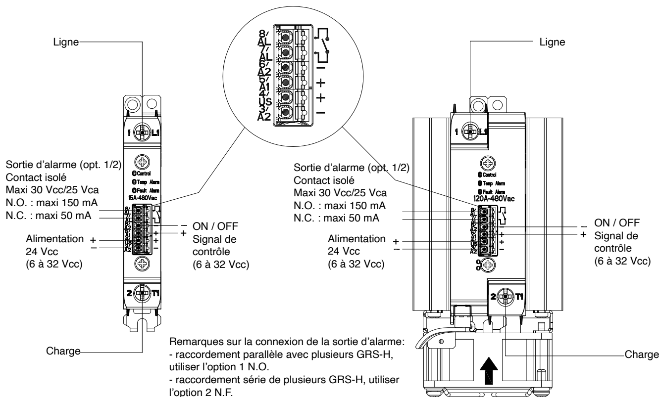
Exemple de raccordement pour GRS-H avec commande Vcc avec option de sortie d'alarme par contact isolé (Options 1 et 2)
