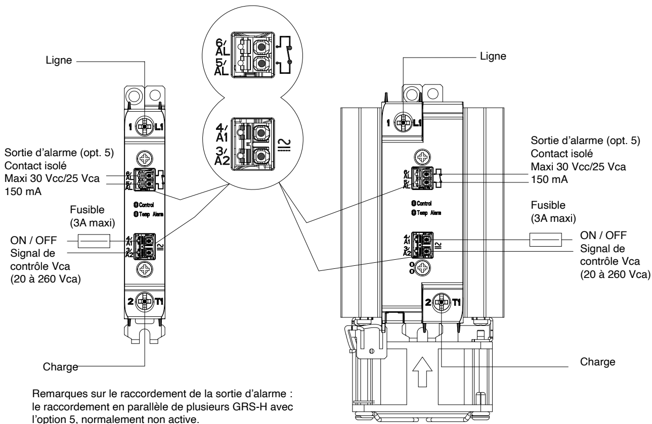
Exemple de raccordement pour GRS-H avec commande Vca avec option d'alarme thermique (Option 5)
