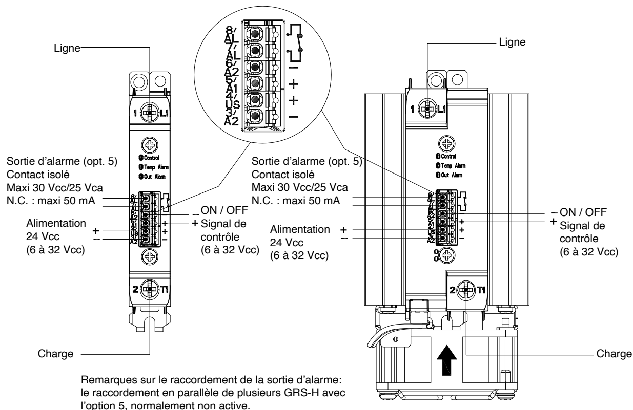
Exemple de raccordement pour GRS-H avec commande Vcc avec option d'alarme thermique (Option 5)
